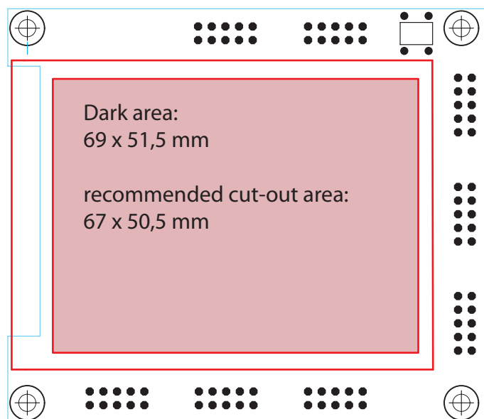
PCB: display side
